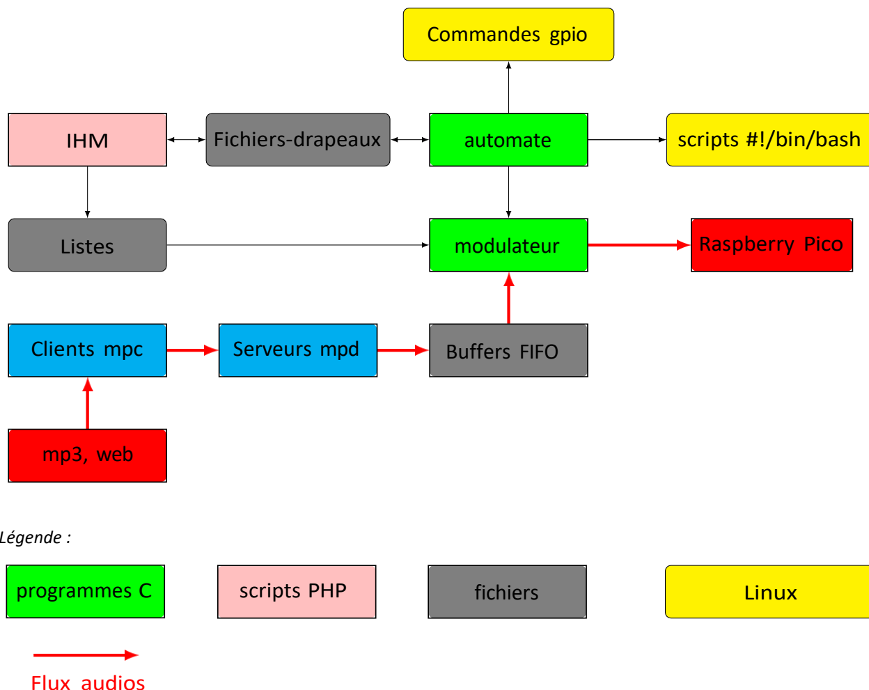
Figure VII-14 : architecture logicielle et flux des données.
