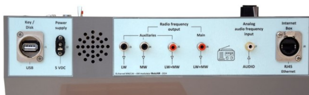
Figure II-06 : face arrière du boîtier d'accueil supportant l'ensemble de la connectique des entrées et sorties.
