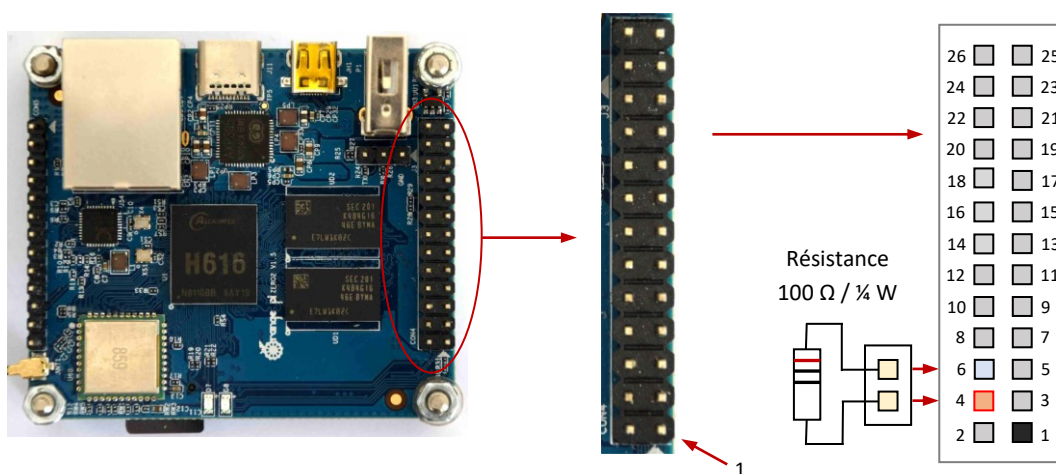
Figure VII-13 : raccordement d'une résistance de décharge de l'alimentation.
