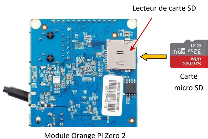
Figure III-7 : insertion de la carte mémoire micro SD 32 Go dans le lecteur du module OPZ.
