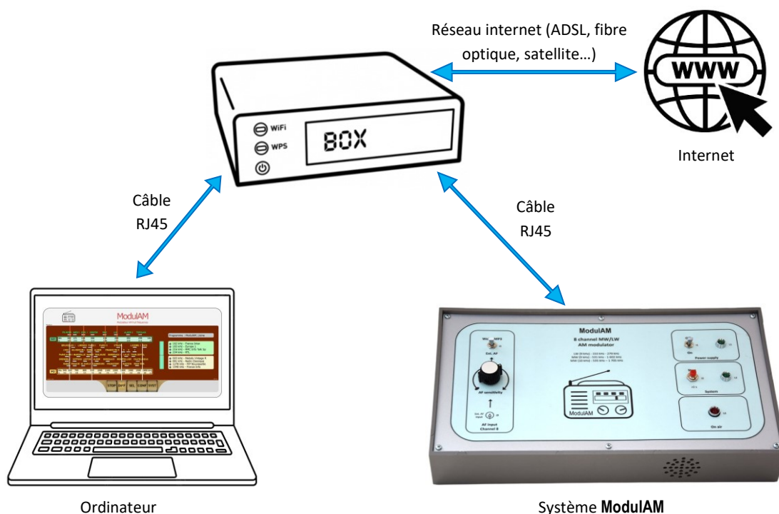
Figure VI-1 : principe de raccordement du ModulAM pour une exploitation à partir du logiciel IHM de configuration avancée et d'édition des stations, des fréquences et des flux audio de modulation, via le réseau local personnel d'une installation classique d'accès à l'internet.
