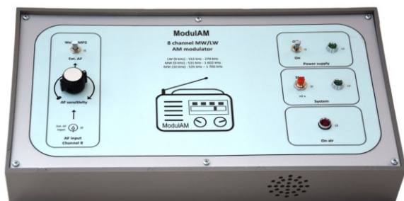
Figure II-05 : face avant du boîtier d'accueil supportant les commandes et signalisations.
